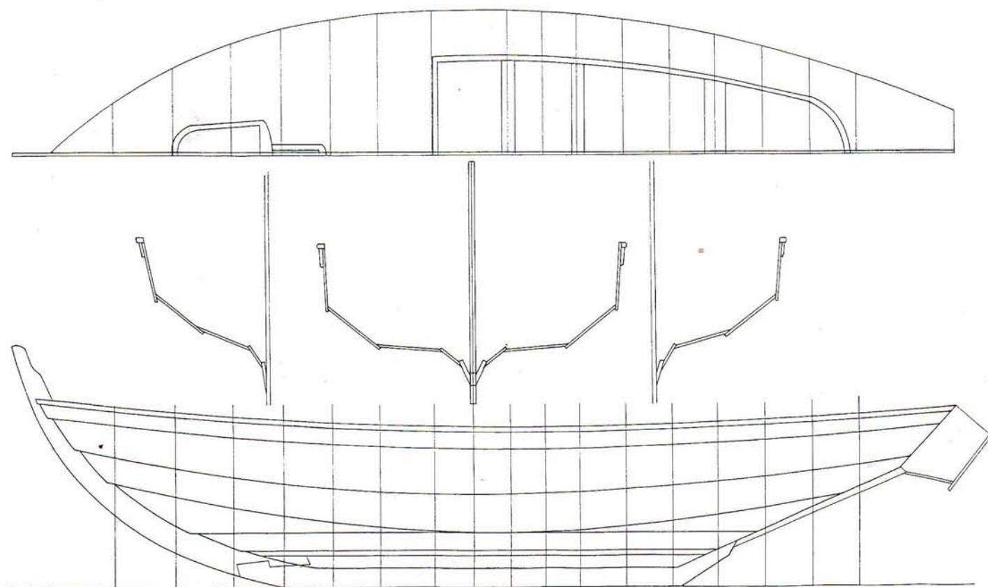
PLANO DE CONSTRUCCION DA DORNA MECA
